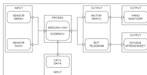
Gambar 3. Rancangan Diagram Blok
