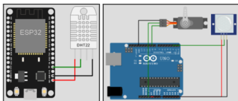
Gambar 4. Rangkaian alat Pemantauan suhu
