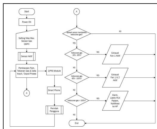
Gambar 2. Flowchart Sistem Kerja Alat
