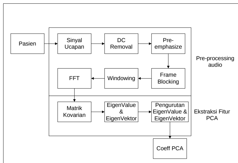
Gambar 2. Blok Diagram PCA
