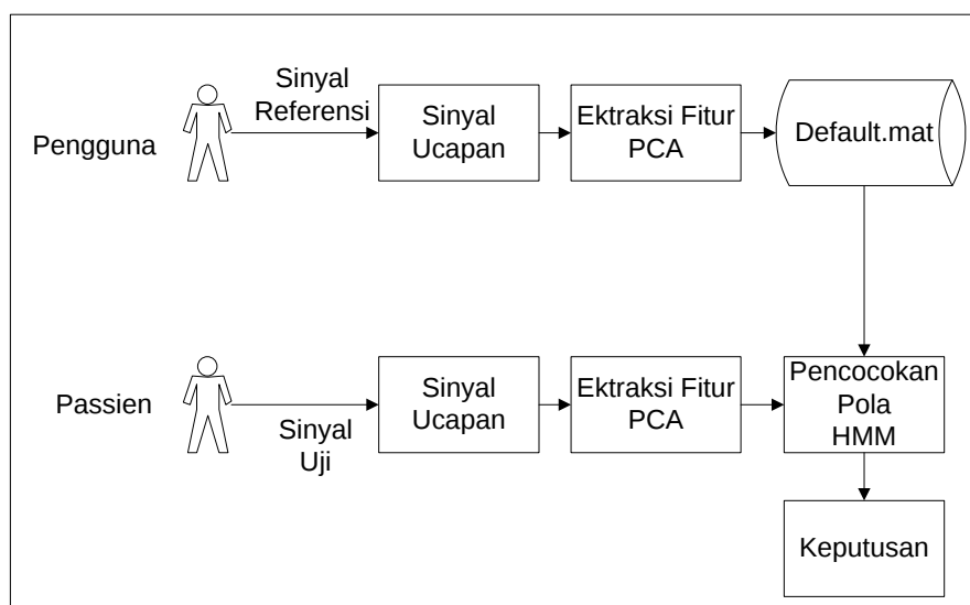
Gambar 1. Sistem Kerja Aplikasi Pengenalan Ucapan
