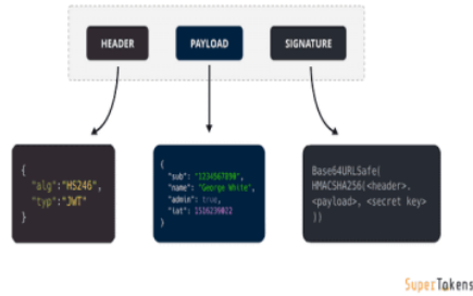
Gambar 1 Bagian JSON Web Token
